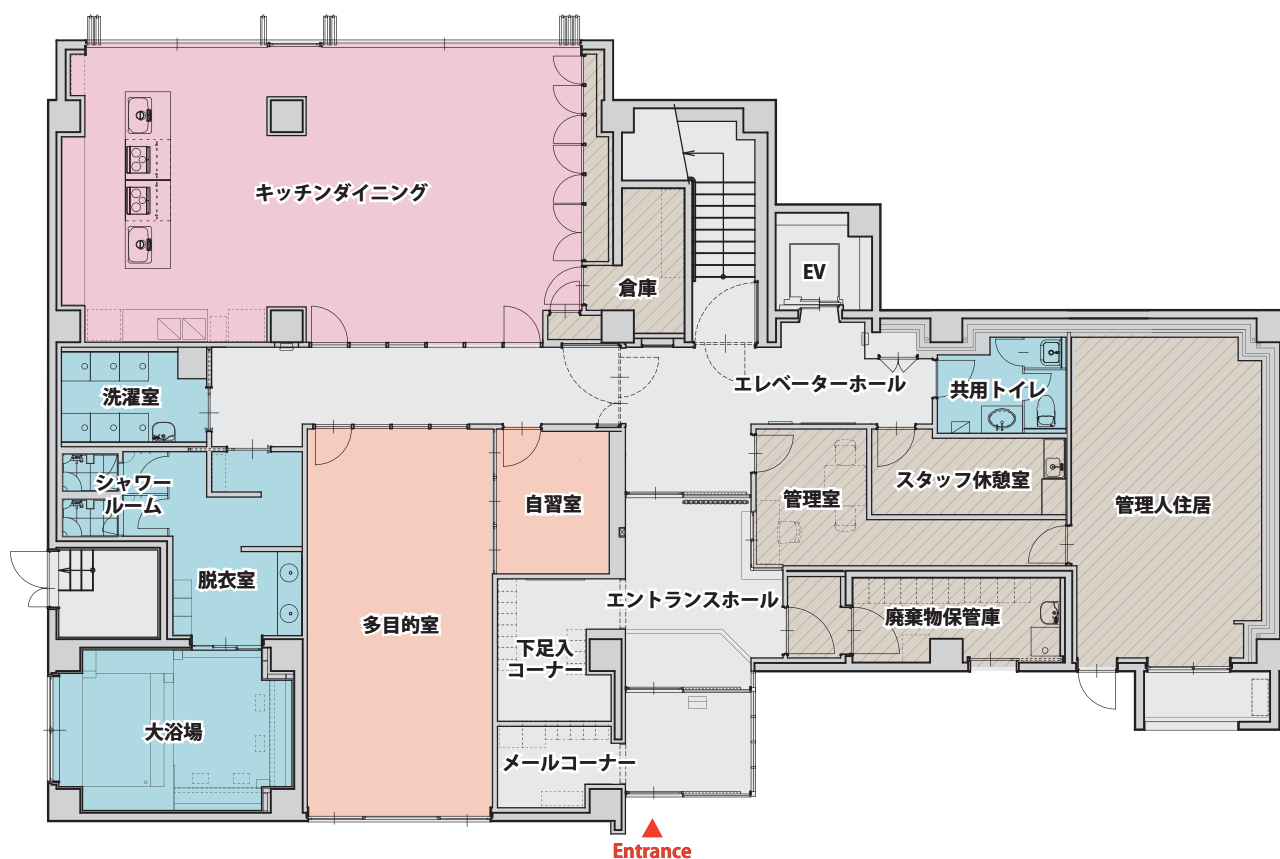
【1階 平面図】
